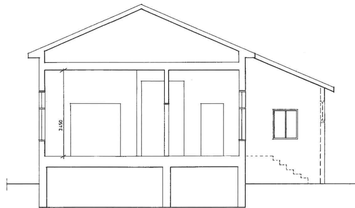
LEIKKAUS A-A
